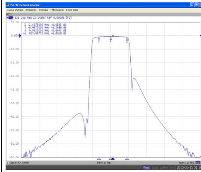
Ripple
