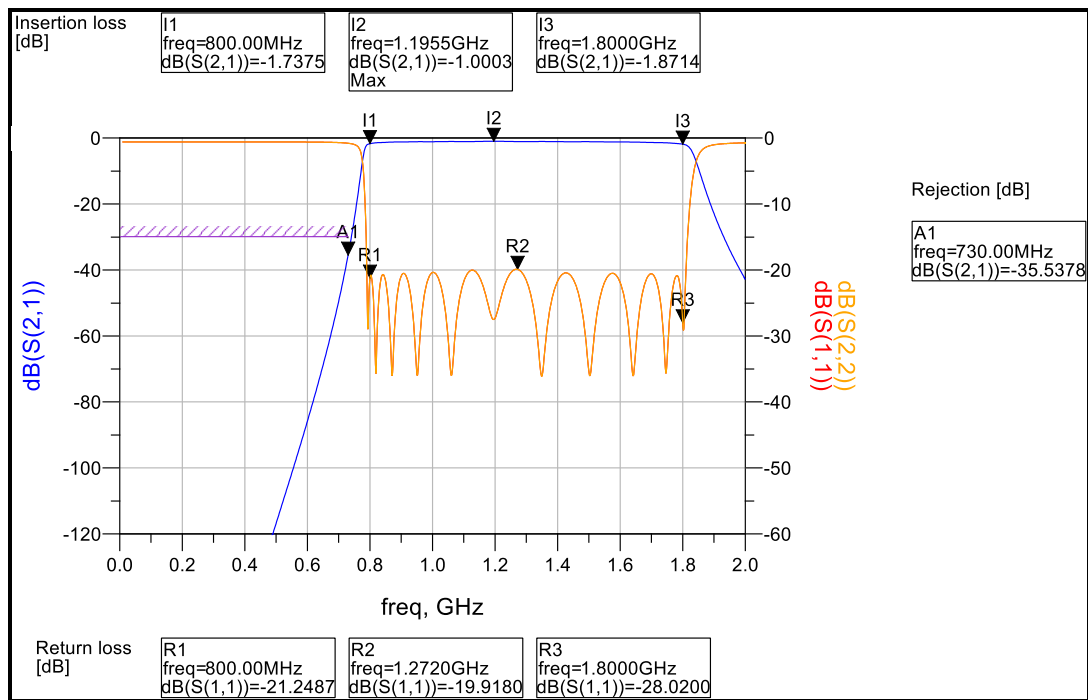
S-parameter
